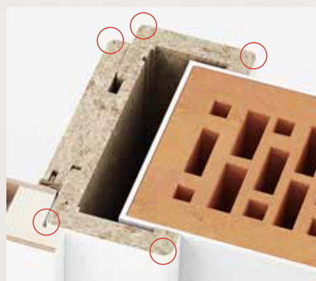
SMS Umfassungszarge mit gerundeten Bekleidungen und gerundetem Futterbrett
