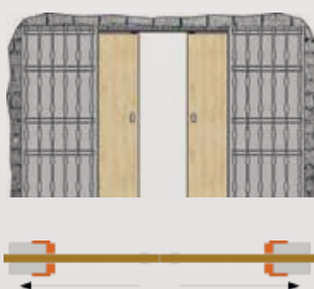
2-FLÜGELIGE AUSFÜHRUNG IN DER WAND LAUFEND
