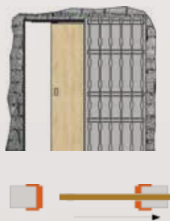
1-FLÜGELIGE AUSFÜHRUNG IN DER WAND LAUFEND
